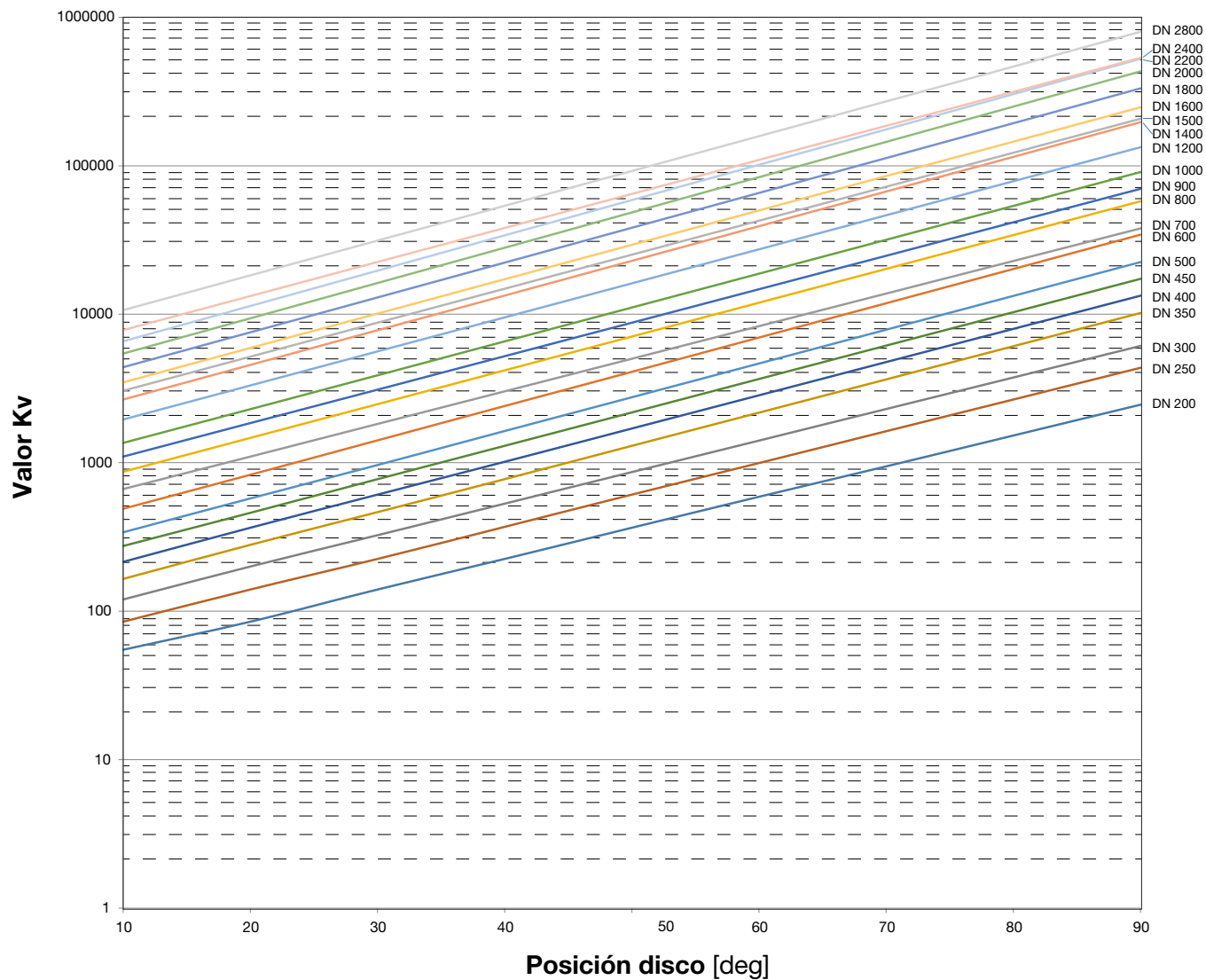
Valores Kv para válvulas de mariposa DN 200 - 2800
