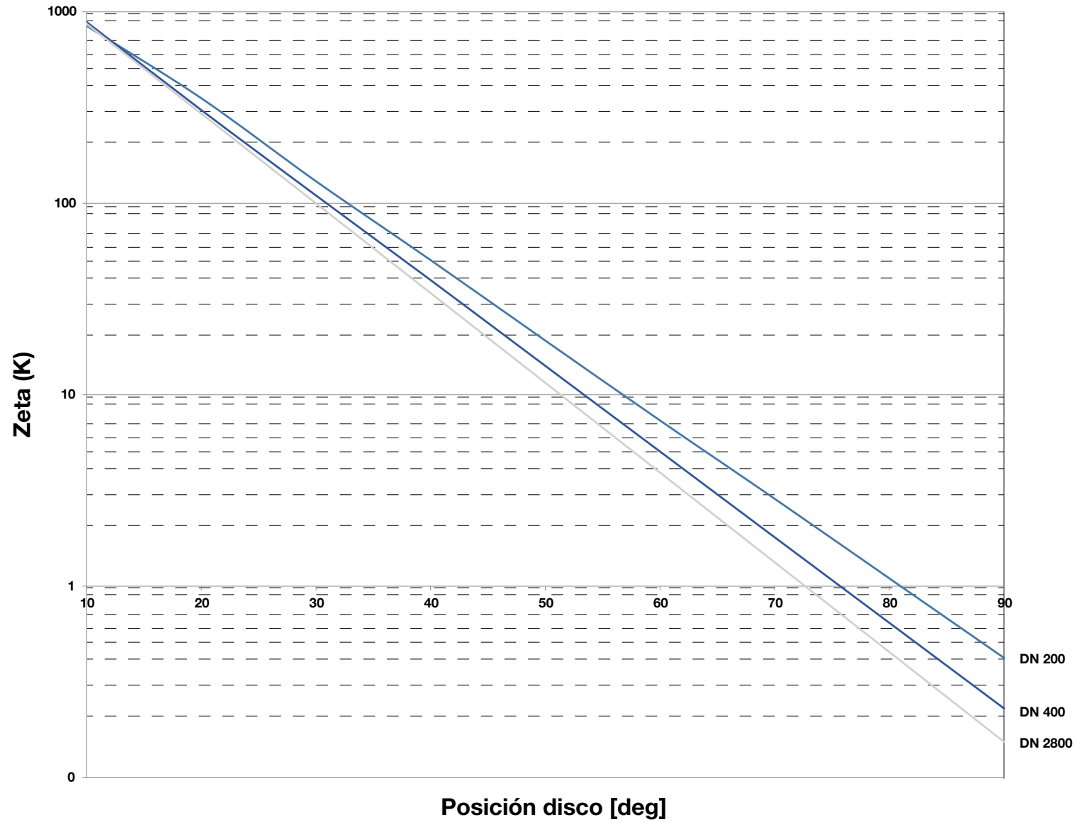
Zeta (K), válvulas mariposa DN 200 - 2800
