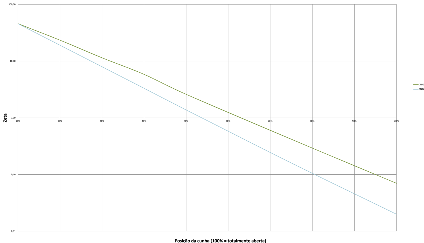
Zeta (K) para válvulas de cunha DN40-DN1200
