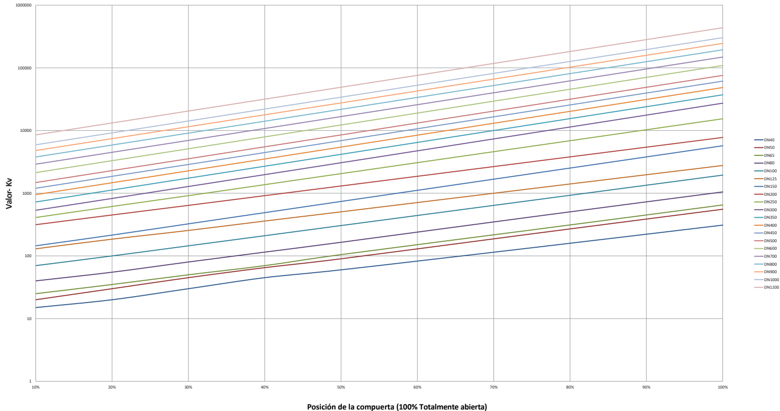
Curva Kv para válvulas de compuerta DN40-DN1200
