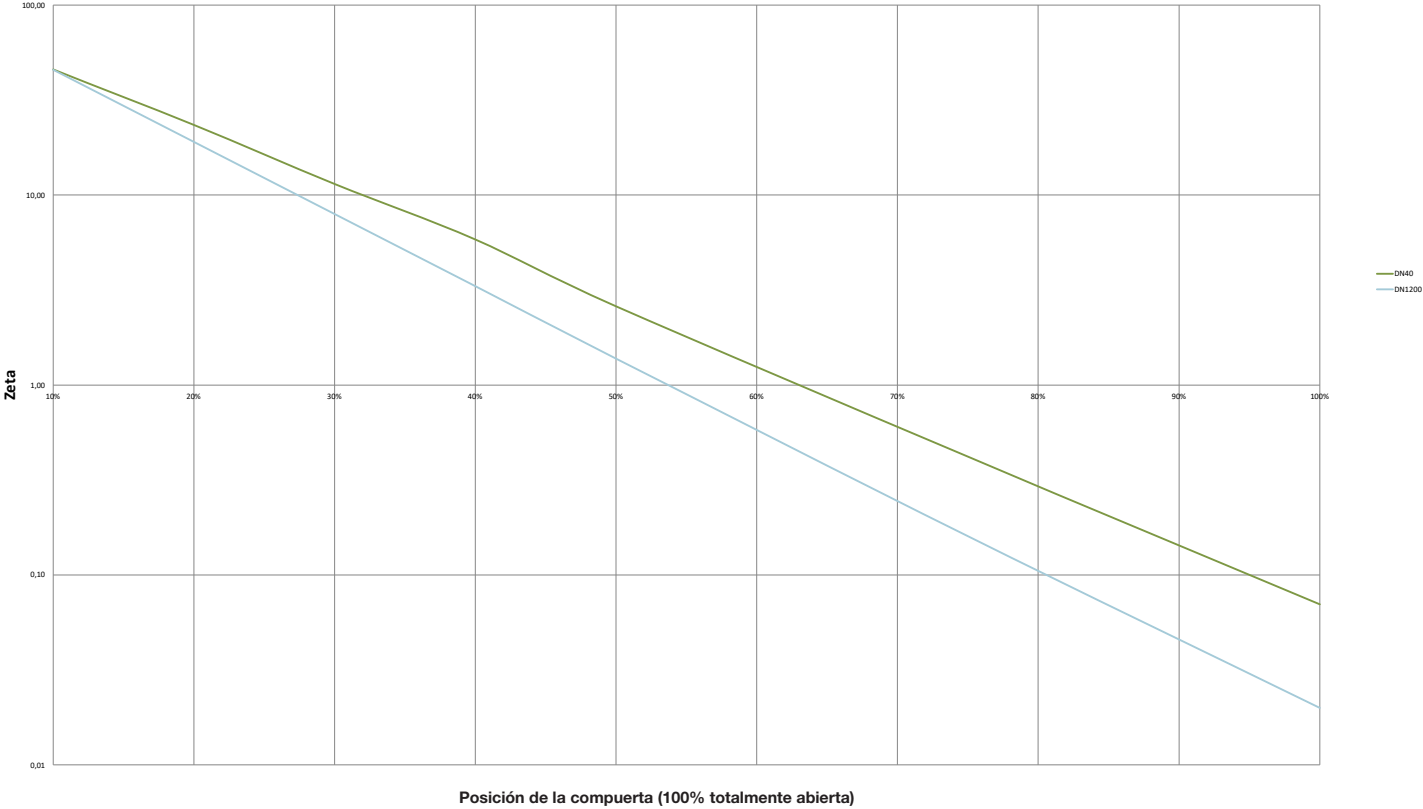
Zeta (K) para válvulas de compuerta DN40 - 1200
