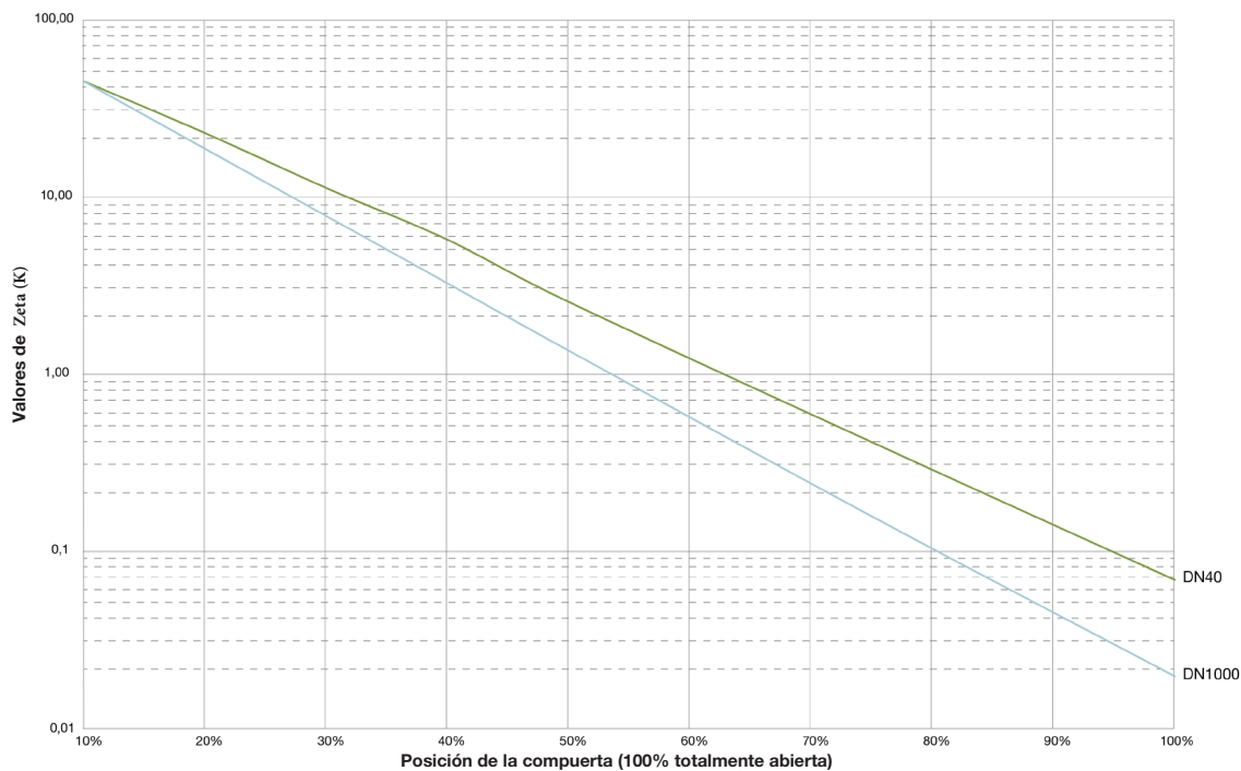
Zeta (K) para válvulas de compuerta DN40 - 1000
