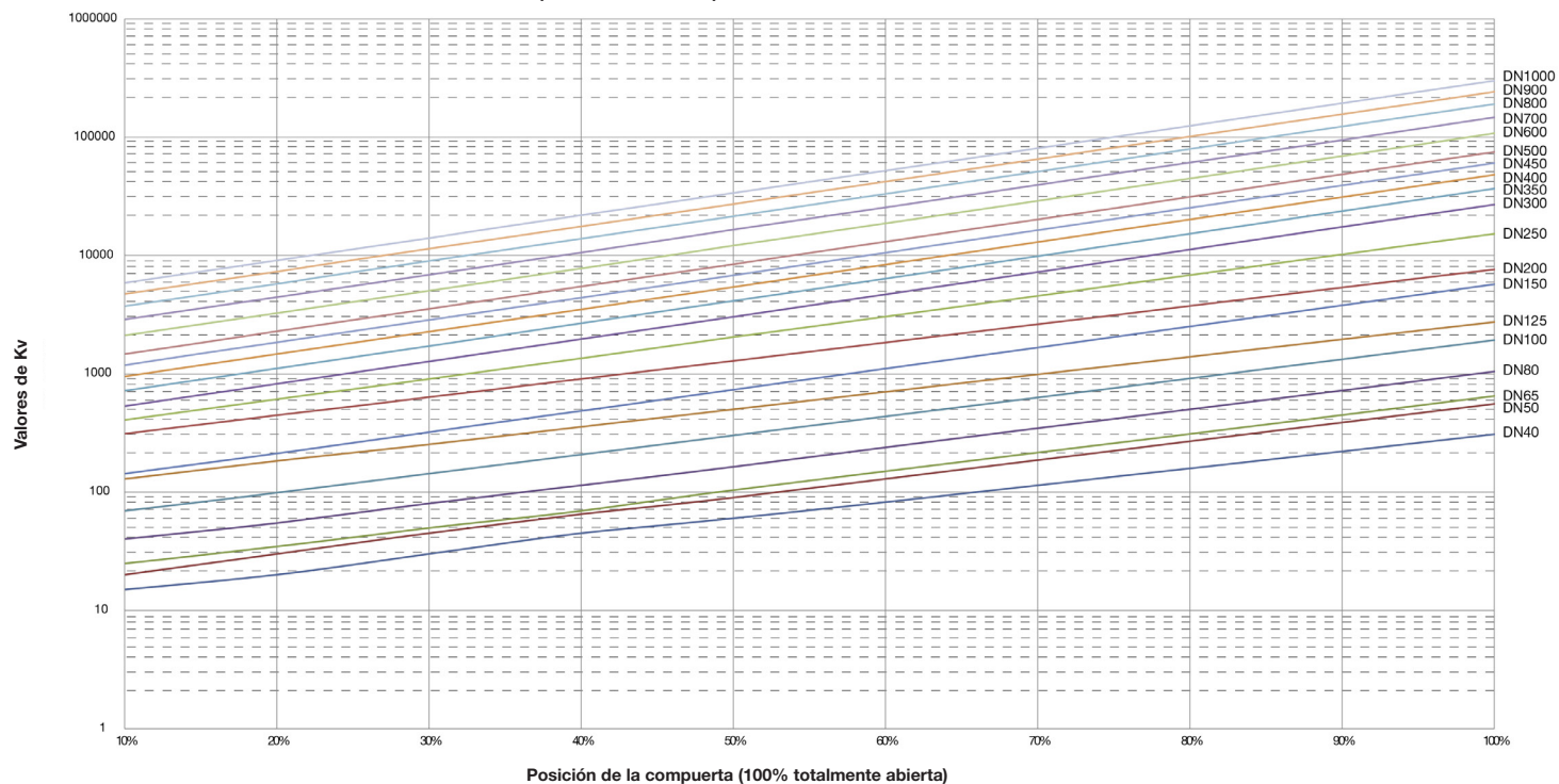
Kv para válvulas de compuerta DN40 - 1000
