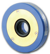
Serie 711 Limitador de flujo, tipo Wafer de limpieza automática con anillo único DN50-200 PN10 Acero carbono Placa latón Caucho NBR
