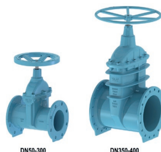
Serie 9002/60 Válvula de compuerta embridada EN 558/15 largo DN50-400 PN10/16 Fundición dúctil Eje inoxidable Caucho EPDM
